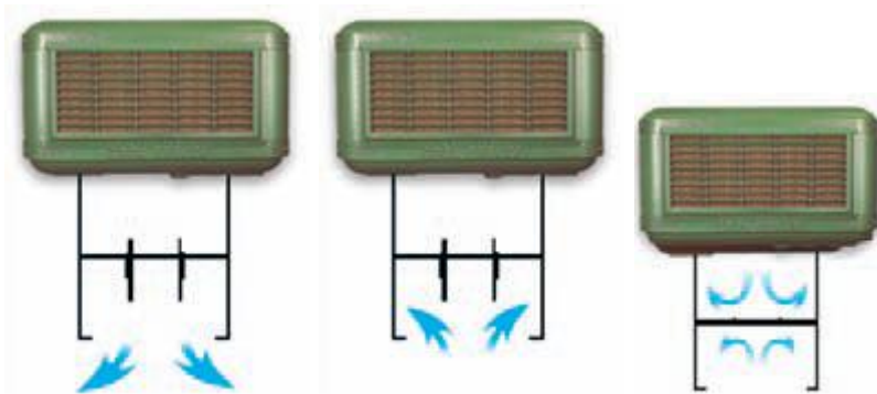
Climatización, Extracción Cerrado Salidas Verticales
